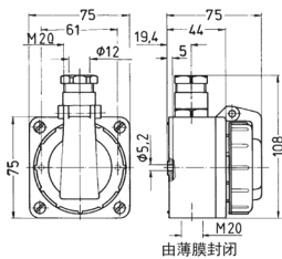
图纸 1MB 347 尺寸毫米
